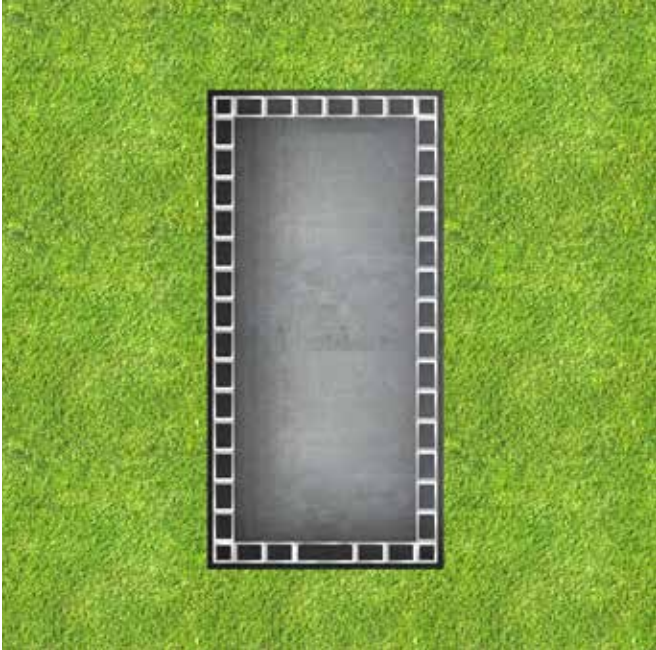
a sx: scavo per piscina tradizionale (500x900 cm.) a dx: scavo per piscina ModoPool® (400x800 cm.)
